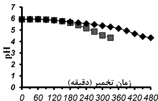
شکل ۱- اثر نوع باکتری بر تغییرات pH در تخمیر (دما ۳۷°C):
