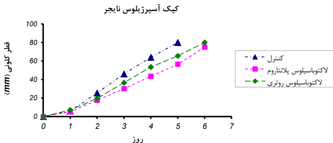
شکل ۳- منحنی رشد کپک اسپرژیلوس نایجر در حضور و عدم حضور مایع‌های رویی حاصل از دو نوع خمیرترش در طی ۶ روز در دمای ۲۵ درجه سانتی‌گراد
