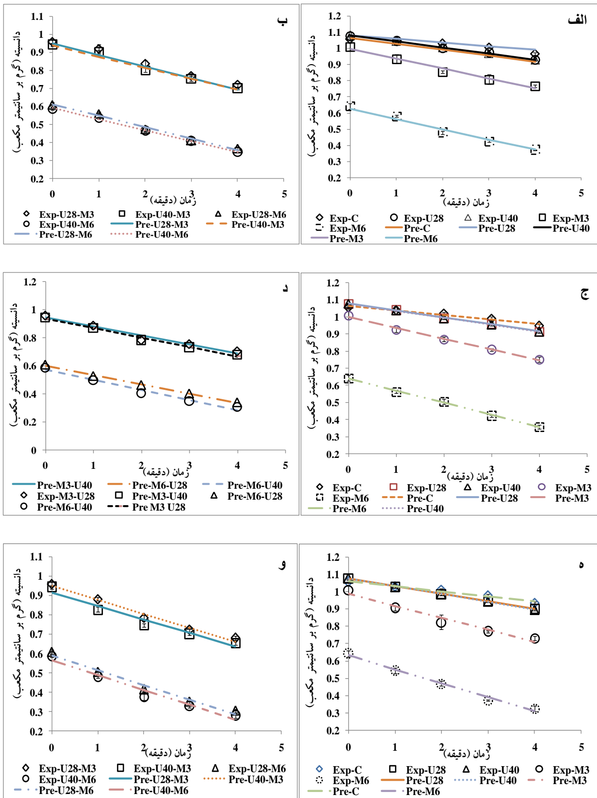
شکل ۲- دانسیته ظاهری قطعات سیب‌زمینی سرخ‌شده حاصل از آزمایش (Exp) و برازش شده (Pre) با مدل ۱ جدول ۶ در ماه‌های ۱۵۰ (الف، ب)، ۱۷۰ (ج، د) و ۱۹۰ (ه، و) درجه سانتی‌گراد در پیش‌تیمارهای مختلف بر اساس جدول ۱
