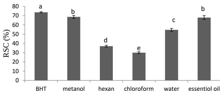
شکل ۴- مقایسه اثر مهارکنندگی رادیکال های آزاد (%) هر عصاره در مقایسه با BHT
