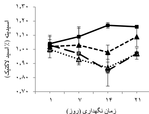
شکل ۳- تغییرات اسیدیته در طول دوره‌ی نگهداری در دمای ۴ °C
