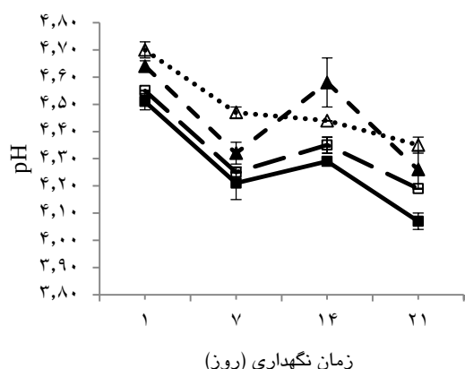
شکل ۲- تغییرات pH در طول دوره‌ی نگهداری در دمای ۴°C (Δ) نمونه‌ی شاهد، (▲) نمونه‌ی غنی شده با ایزوله‌ی پروتئین سویا، (□) نمونه‌ی تیمار شده با آنزیم ترانس گلوتامیناز، (■) نمونه‌ی تواما غنی شده با ایزوله‌ی پروتئین سویا و تیمار شده با آنزیم ترانس گلوتامیناز.
