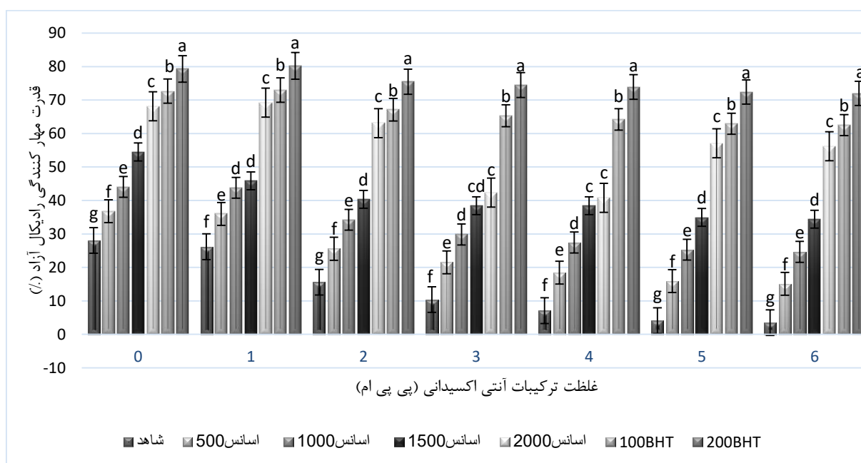
شکل ۳- نمودار فعالیت مهارکنندگی DPPH (پی پی ام) مایونز با اسانس ترخون در طول دوره‌ی شش‌روزه (۰، ۵۰۰، ۱۰۰۰، ۱۵۰۰ و ۲۰۰۰) در مقابل آنتی‌اکسیدان سنتزی BHT (۱۰۰ و ۲۰۰)
