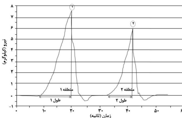
شکل ۱- منحنی تیپیک نیرو به زمان دو مرحله فشرده‌سازی ژل سوریمی ماهی شوریده دهان سیاه جهت تعیین پارامترهای ساختار بافت
