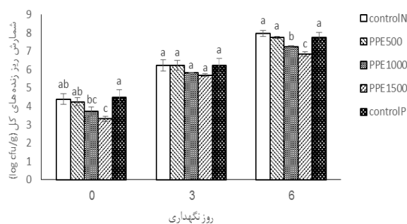
شکل ۲- شمارش کلی باکتری‌ها ( \log \text{cfu/g} ) نمونه‌های
